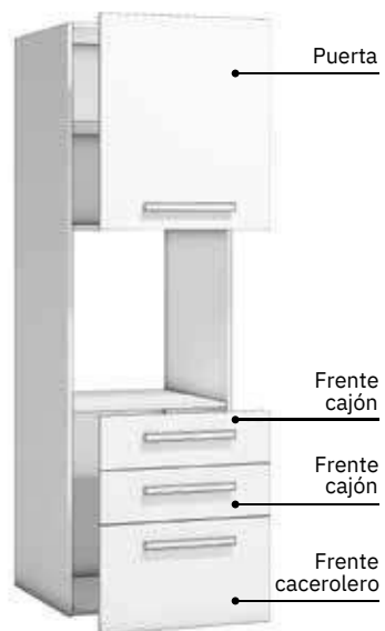
Mueble Columna Horno 1 puerta/2 cajones/1 cacerolero
